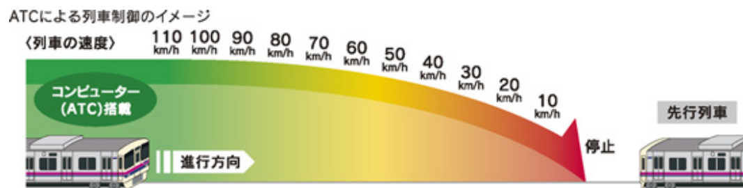
《ATCによる列車制御のイメージ》
